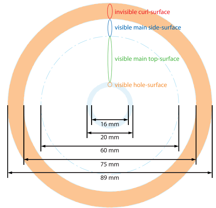
Dimensioning
